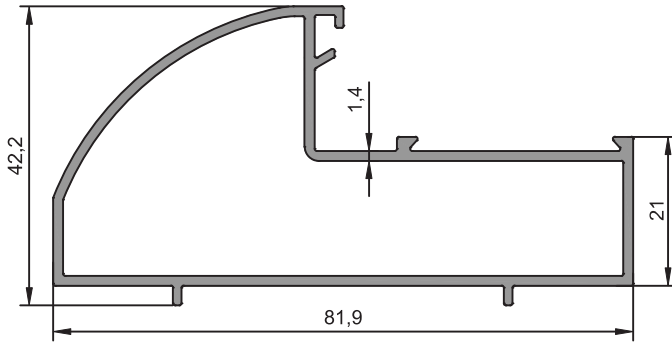
2925 Kapı Kasa Profili 1,297 kg/m
