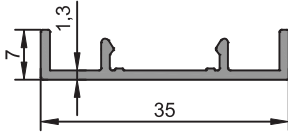
2921 Kapak Profili 0,196 kg/m
