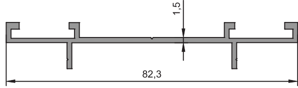
2944 Bağlantı Profili 0,670 kg/m
