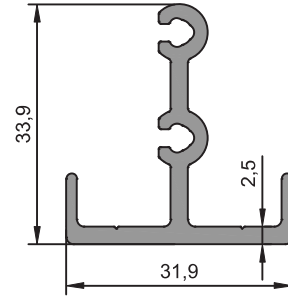
2920 Bağlantı Profili 0,503 kg/m
